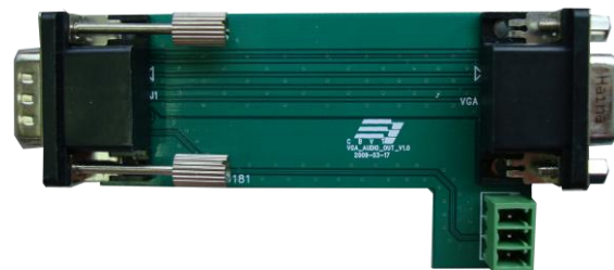
The VGA insert module
